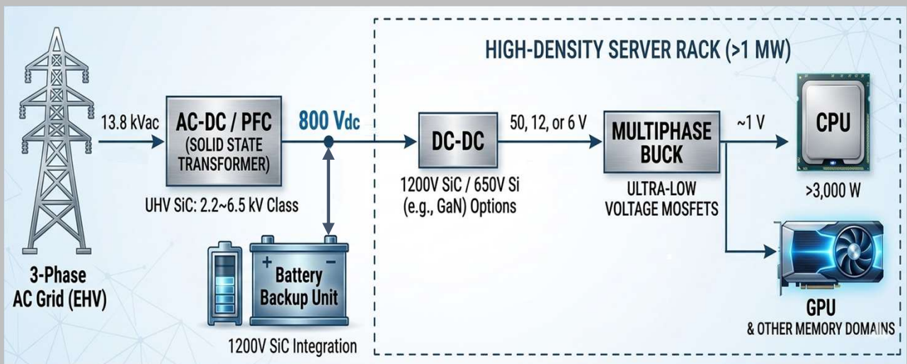
電力管理システム: 800V配電から中間バスおよび低圧盤レールまで
