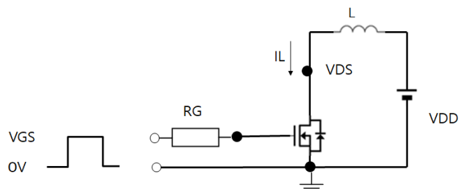
図2 測定回路例
