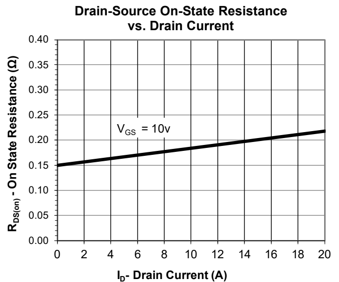
図13 I_D - R_{DS(ON)} 特性
